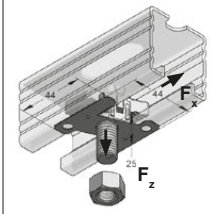
Stex 45 płytka montażowa z bolcem MTB
